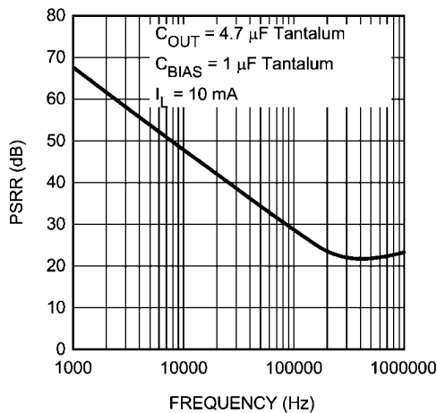
V_{IN} PSRR
